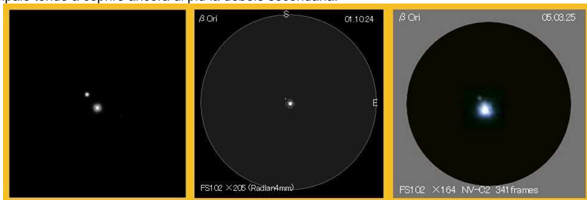
A sinistra, rappresentazione di Beta Orionis attraverso il software Aberrator, al centro un disegno con un telescopio da 102 mm eseguito da Kenichi Kushida a 205x, a destra un'immagine fotografica dello stesso autore che rende evidente come la secondaria sia sommersa dalla luminosità della principale
